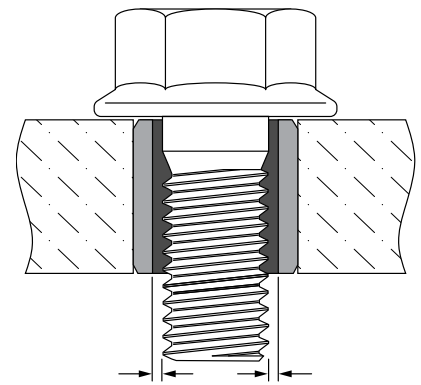
螺栓直径周围的最小间隙为1mm
